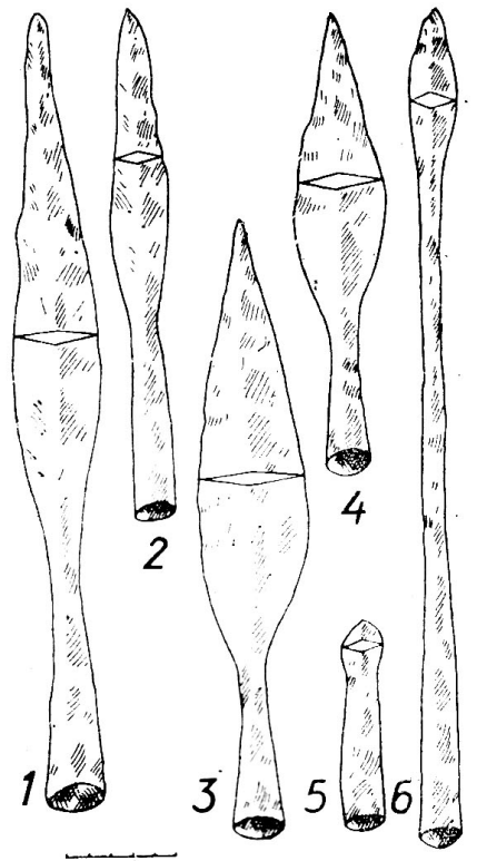
2 pav. Jauneikių kapinyno ietigaliai. 1, 2 — karklo lapo formos plunksnomis (k. Nr. 294), 3, 4 — lauro lapo formos plunksnomis (k. Nr. 466), 5, 6 — rombo formos plunksnomis (k. Nr. 390, 135)
